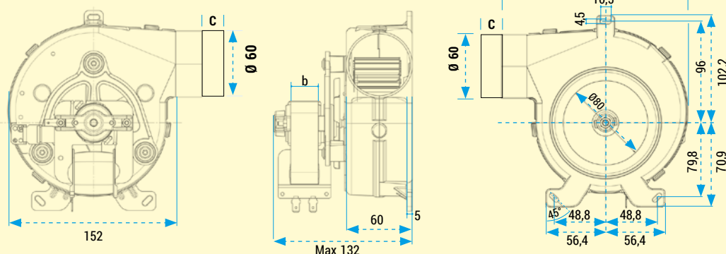
Côté pour déterminer la position du moteur
