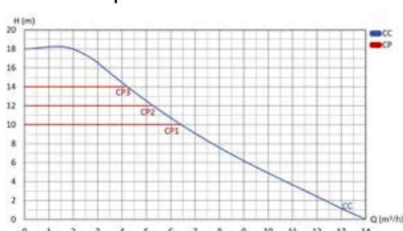
Curve di prestazione Art. P.078.8-
