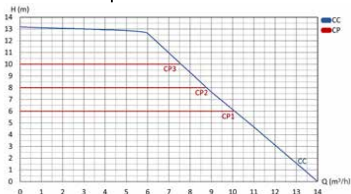
Curve di prestazione Art. P.078.2-
