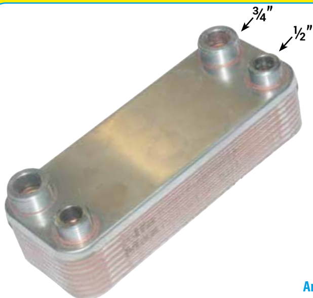
Art. S.004 - Scambiatore "AlfaMax" tipo XS 208 X 75 istantaneo a piastre inox saldobrasate. Attacchi filettati.
