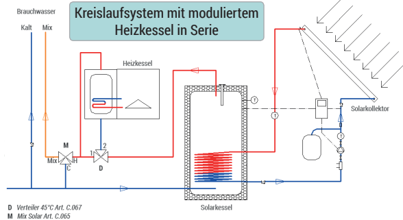
ILLUSTRATIVES INSTALLATIONSSHEMA, NICHT ZUR AUSFÜHRUNG
