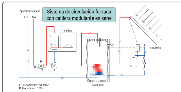
ESQUEMA DE INSTALACION INDICATIVO, A MODO DE EJEMPLO
