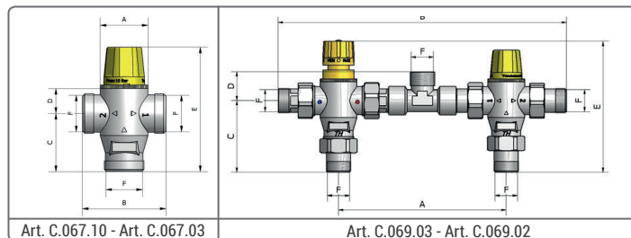
ESQUEMA DE INSTALACION INDICATIVO, A MODO DE EJEMPLO
