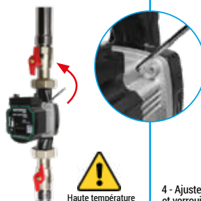
3 - Retirez les boulons hexagonaux avec une clé hexagonale
